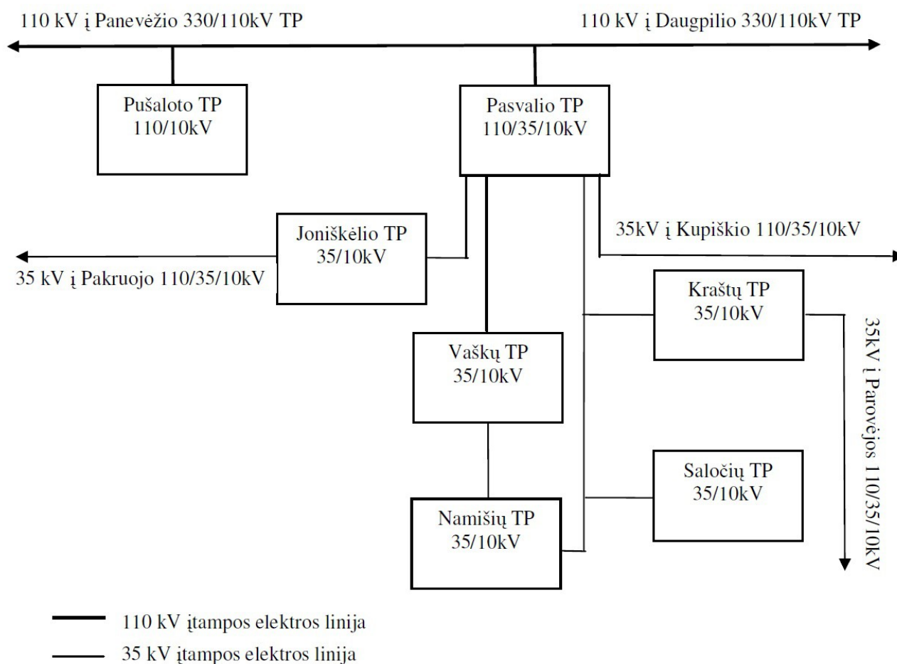
2 pav. Elektros perdavimo ir paskirstymo schema
