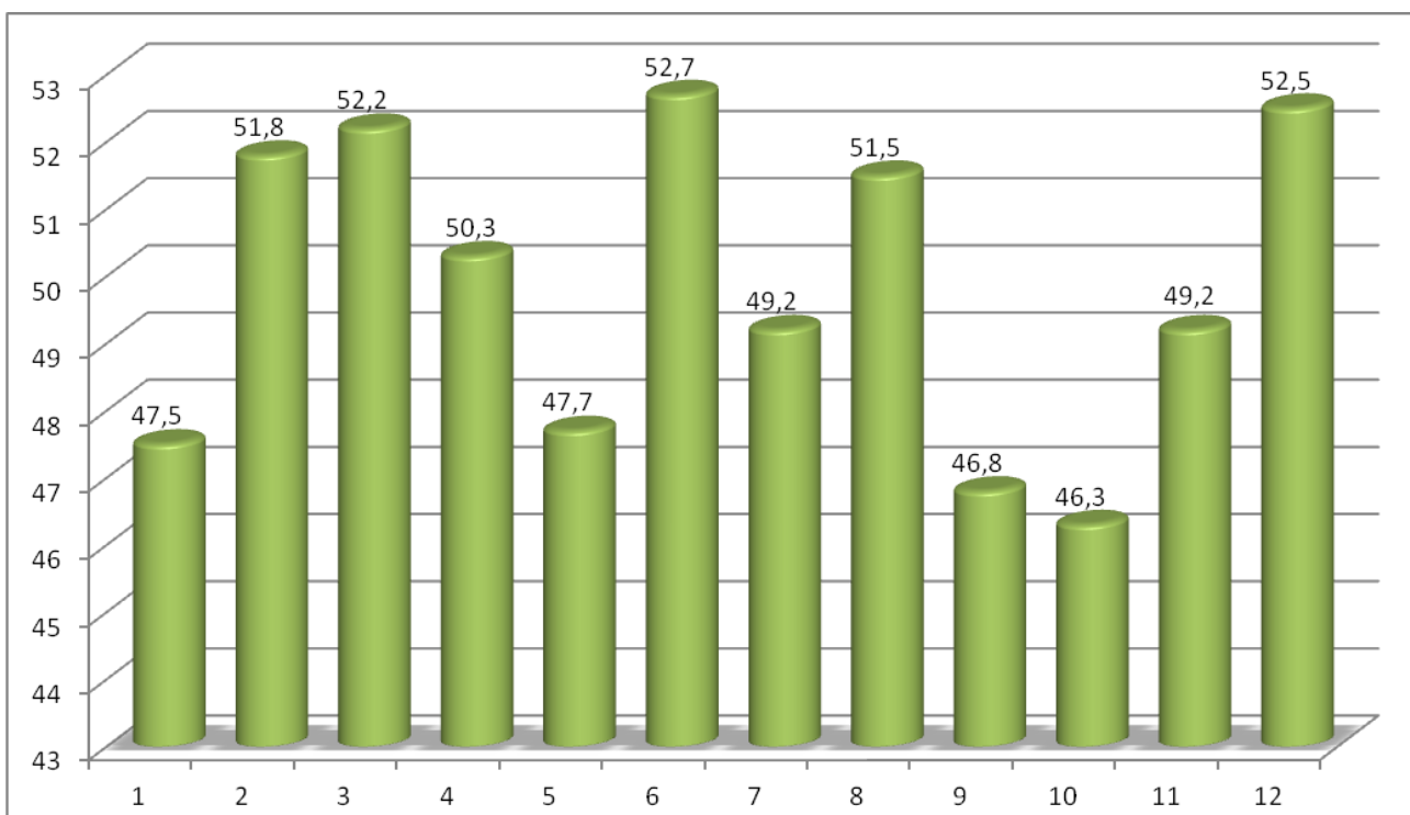
65 pav. Ekvivalentinio triukšmo pasiskirstymas matavimo vietose nakties metu (22-6 val.). Ribinis dydis 55 dBA.
