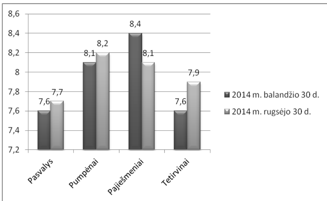
33 pav. pH reikšmė Pasvalio rajono požeminiame vandenyje
