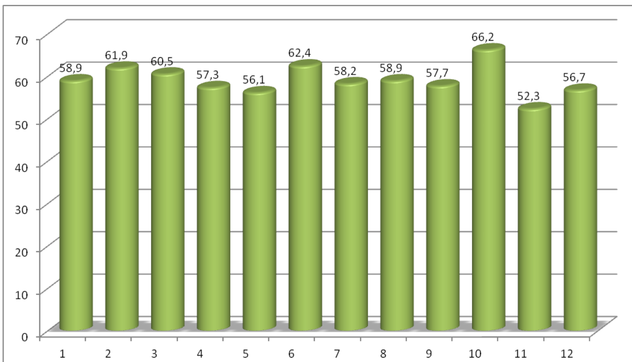
63 pav. Ekvivalentinio triukšmo pasiskirstymas matavimo vietose vakaro metu (18-22 val.). Ribinis dydis 60 dBA.
