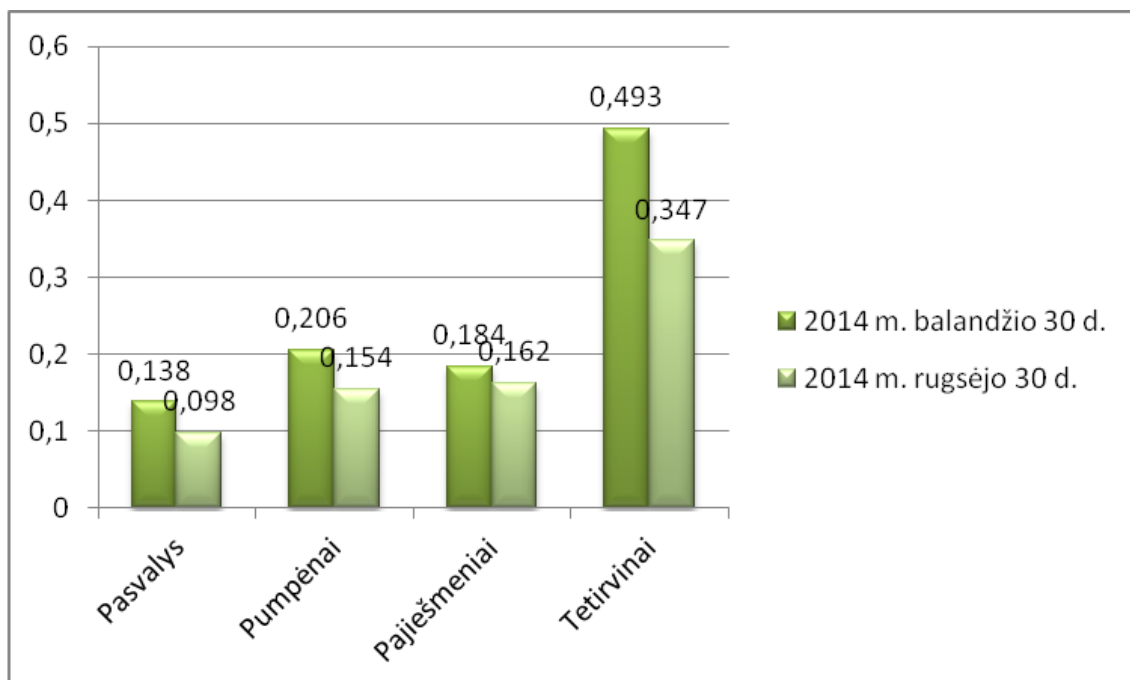
36 pav. Amonio azoto koncentracija Pasvalio rajono požeminiame vandenyje
