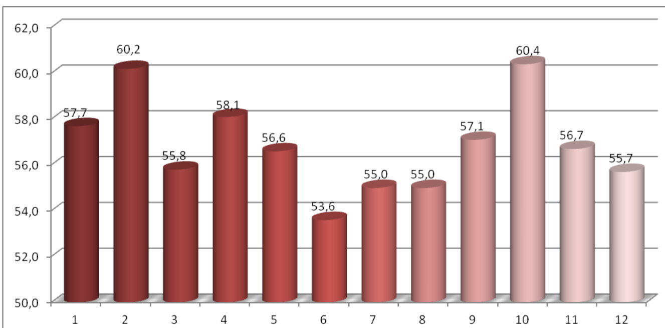
48 pav. Maksimalaus triukšmo pasiskirstymas matavimo vietose nakties metu (22-6 val.). Ribinis dydis 60 dBA.
