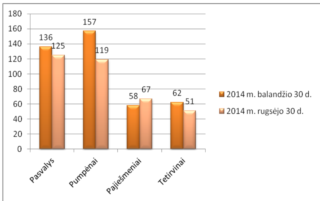
38 pav. Sulfatų koncentracija Pasvalio požeminiame vandenyje
