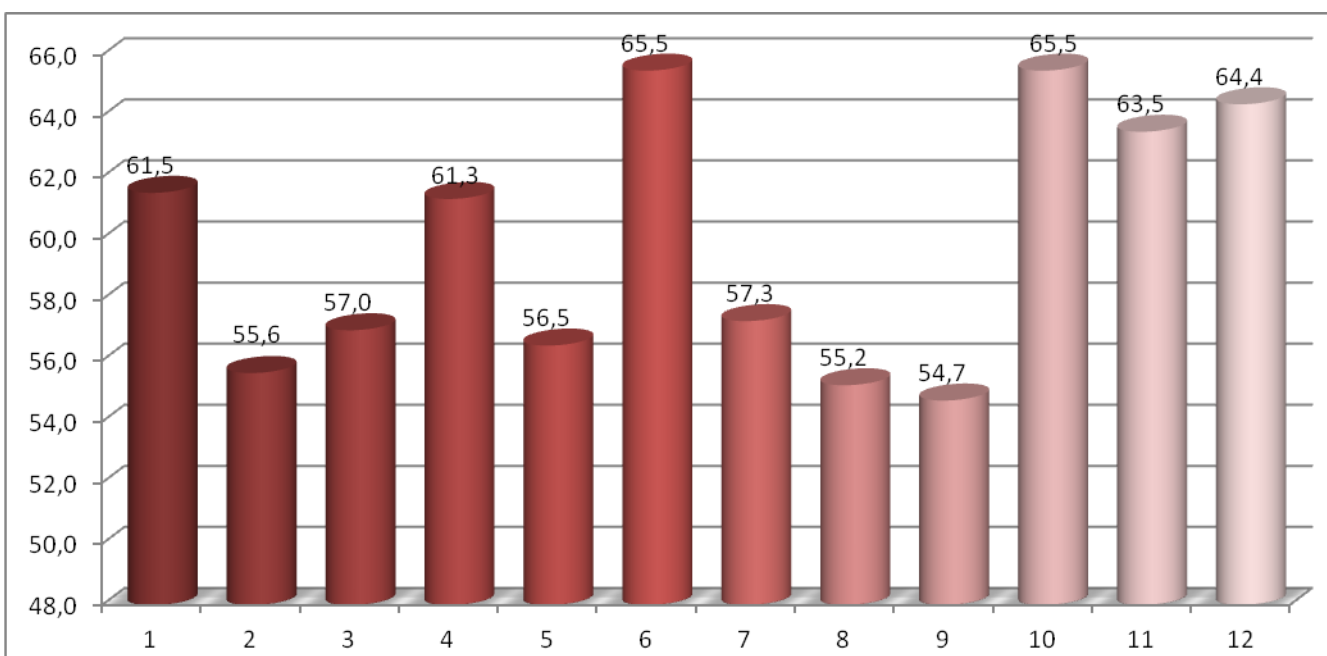
64 pav. Maksimalaus triukšmo pasiskirstymas matavimo vietose nakties metu (22-6 val.). Ribinis dydis 60 dBA.
