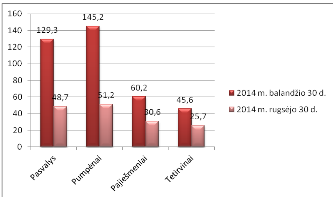
35 pav. nitratų koncentracija Pasvalio rajono požeminiame vandenyje
