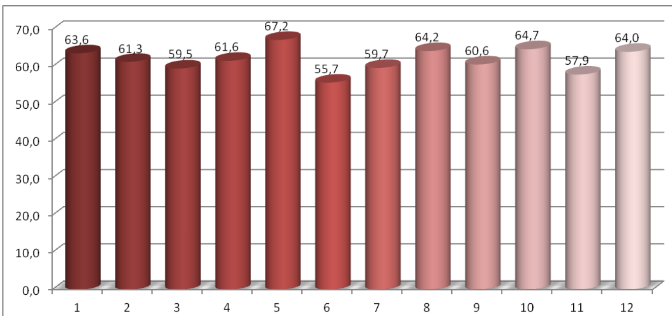
46 pav. Maksimalaus triukšmo pasiskirstymas matavimo vietose vakaro metu (18-22val.). Ribinis dydis 65 dBA.
