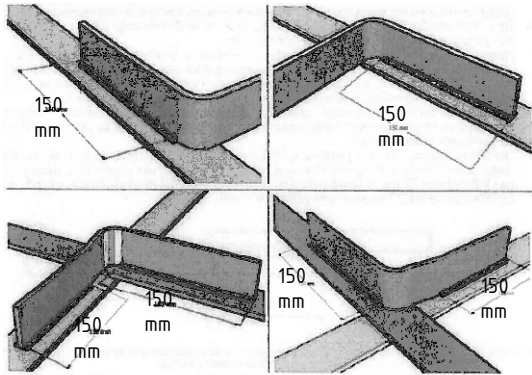
Ižeminimo sistemos stačiakampių profilių jungiamųjų laidininkų suvirinimo elektrolankiniu būdu pavyzdys
