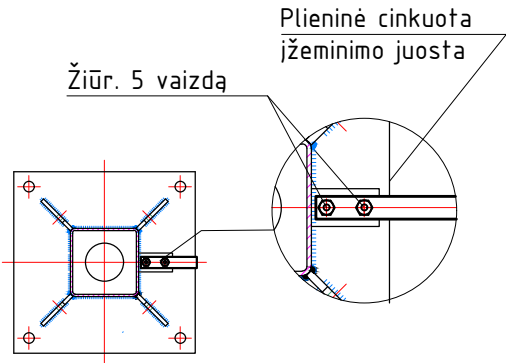
Ižeminimo juostos prijungimas prie metalo konstrukcijų pavyzdys
