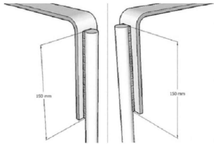
Ižeminimo sistemos apvalaus ir stačiakampių profilių jungiamųjų laidininkų suvirinimo elektrolankiniu būdu pavyzdys
