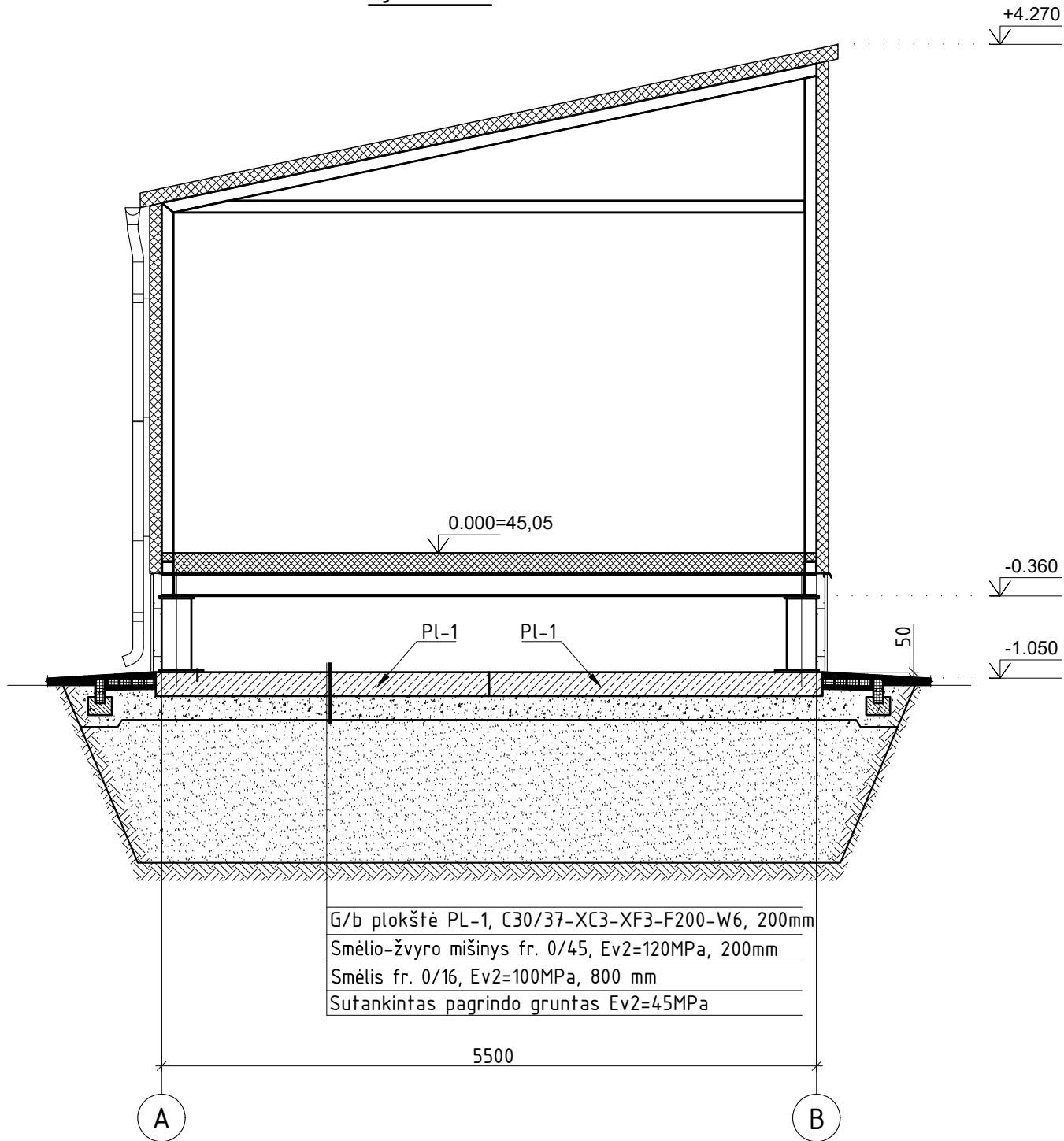
Pjūvis 1-1 M1:50
