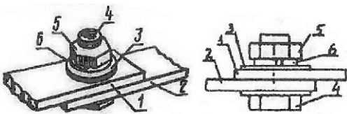
Ižeminimo juostos varžtinis prijungimas prie metalo konstrukcijų pavyzdys
