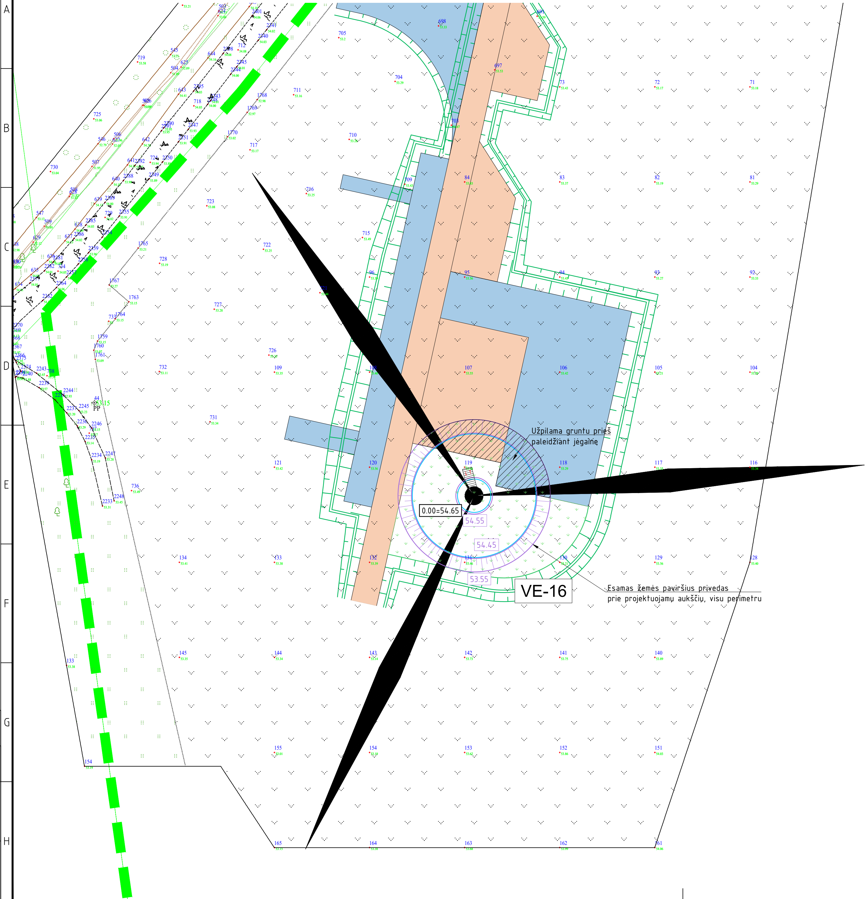
Sklypo aukščių planas M1:500
