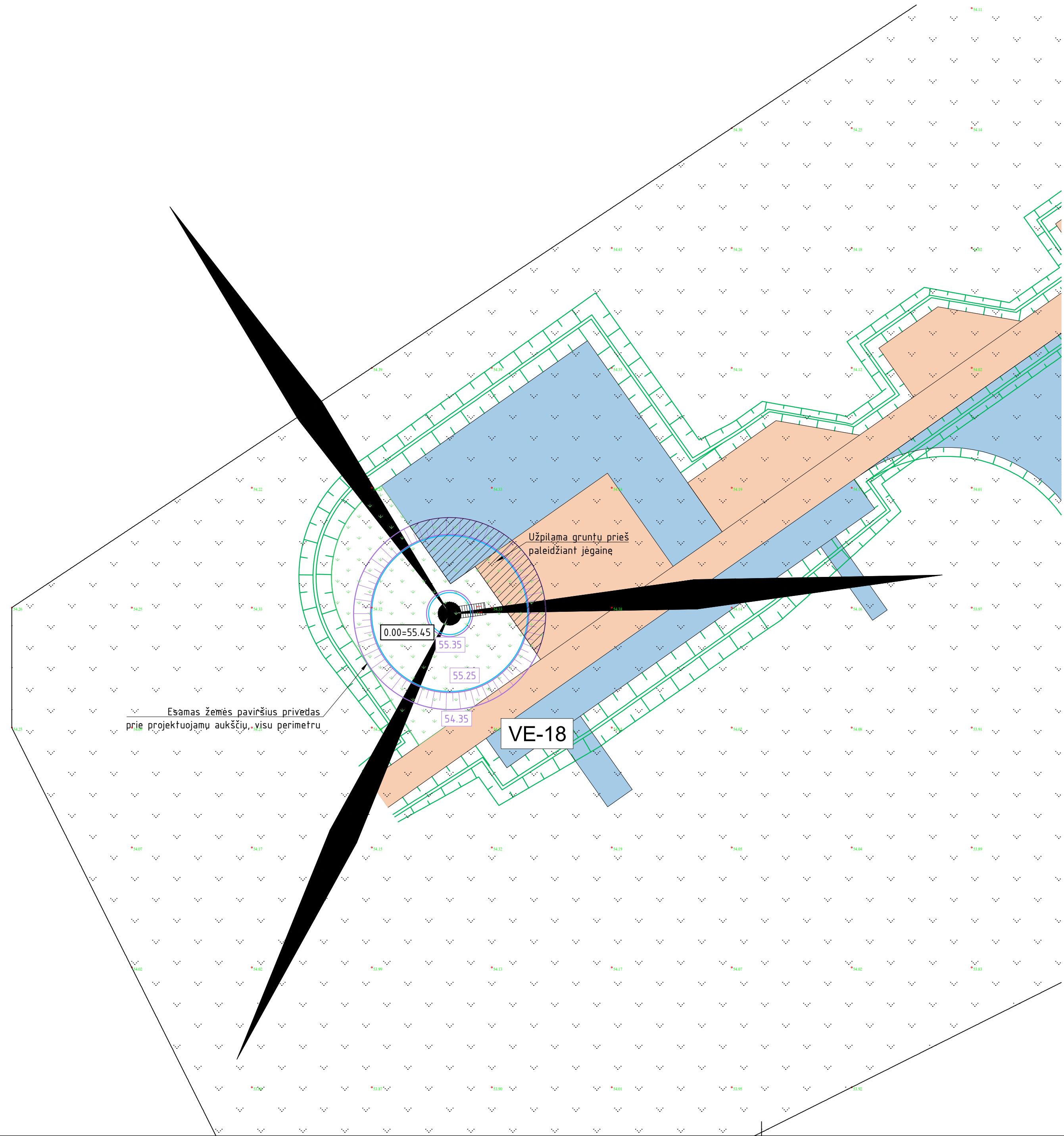
Sklypo aukščių planas M1:500
