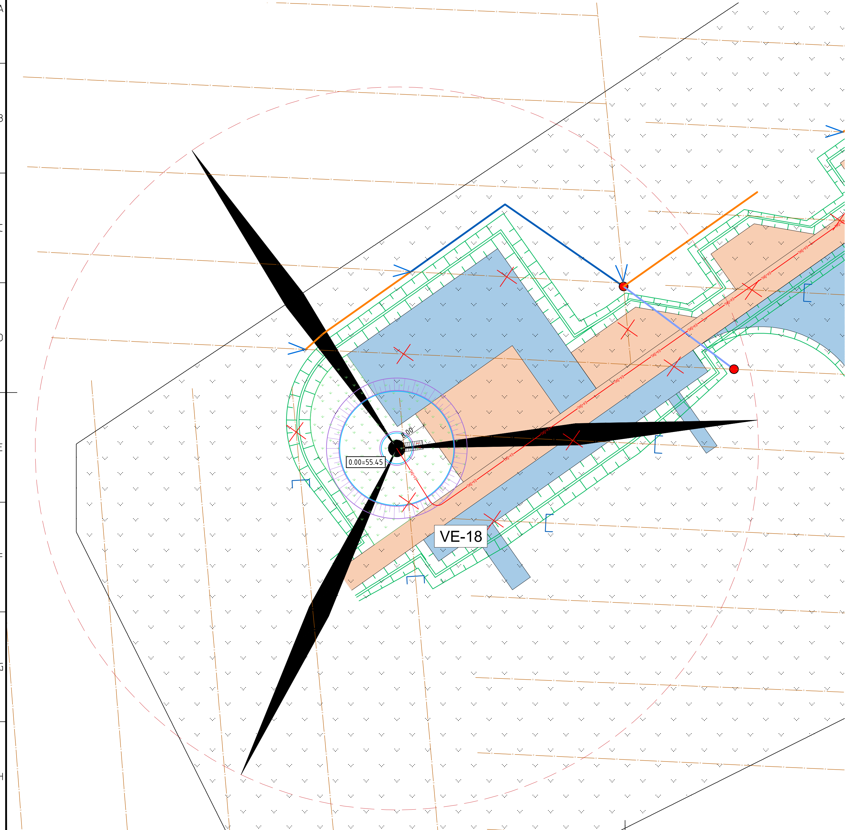
Sklypo planas M1:500
