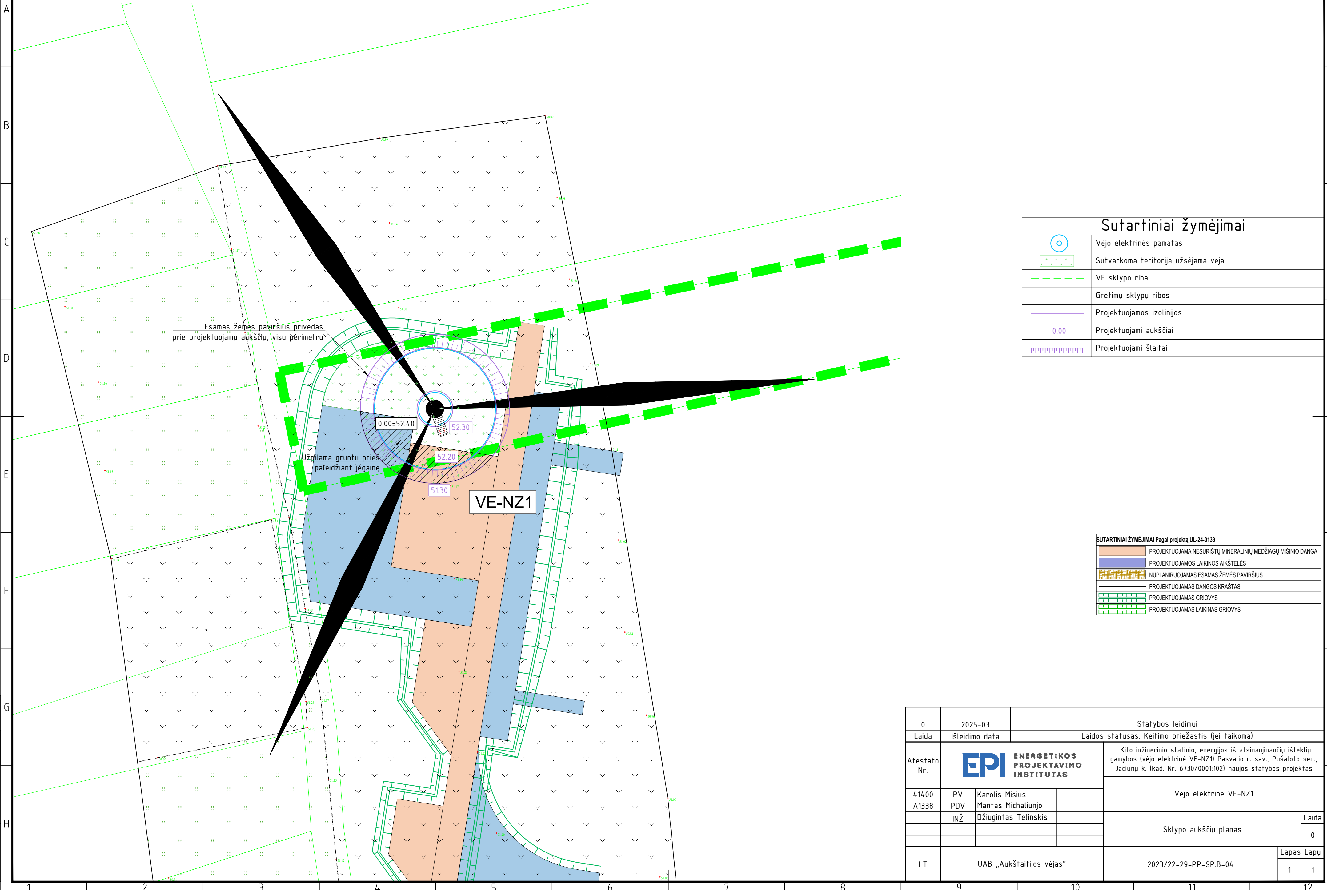
Sklypo aukščių planas M1:500
