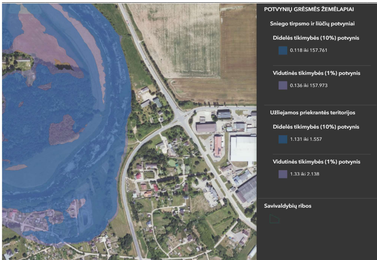
3.6.2 pav. Ištrauka iš Potvynio grėsmės žemėlapio.
