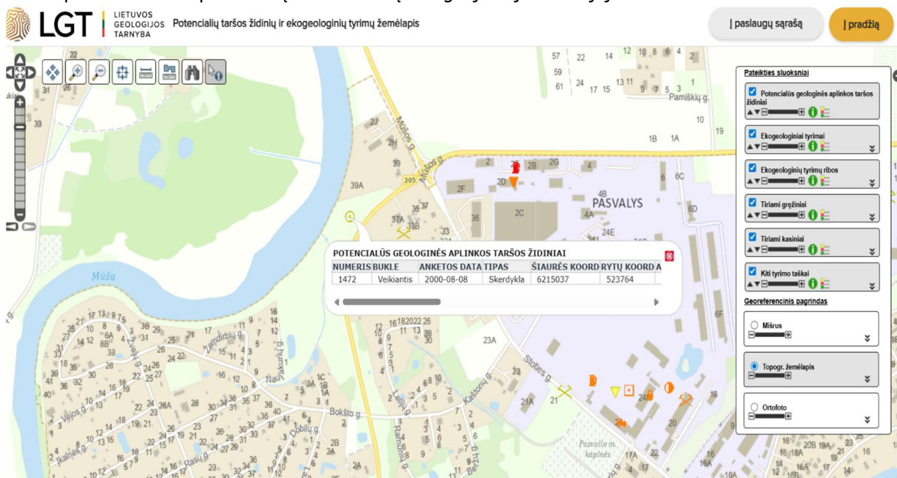
3.6.3 pav. Ištrauka iš Potencialių taršos židinių ir ekogeologinių tyrimų žemėlapio.
