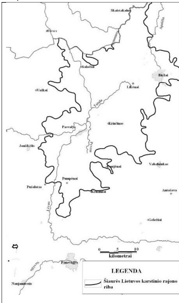
3.6.4 pav. Šiaurės Lietuvos karstinio rajono ribų žemėlapis, 2008 m.
